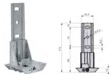
Soporte Inferior
