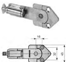
Enganche Superior
